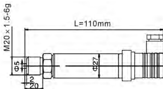
Hirschmann接头型 (M20 × 1.5接口)
