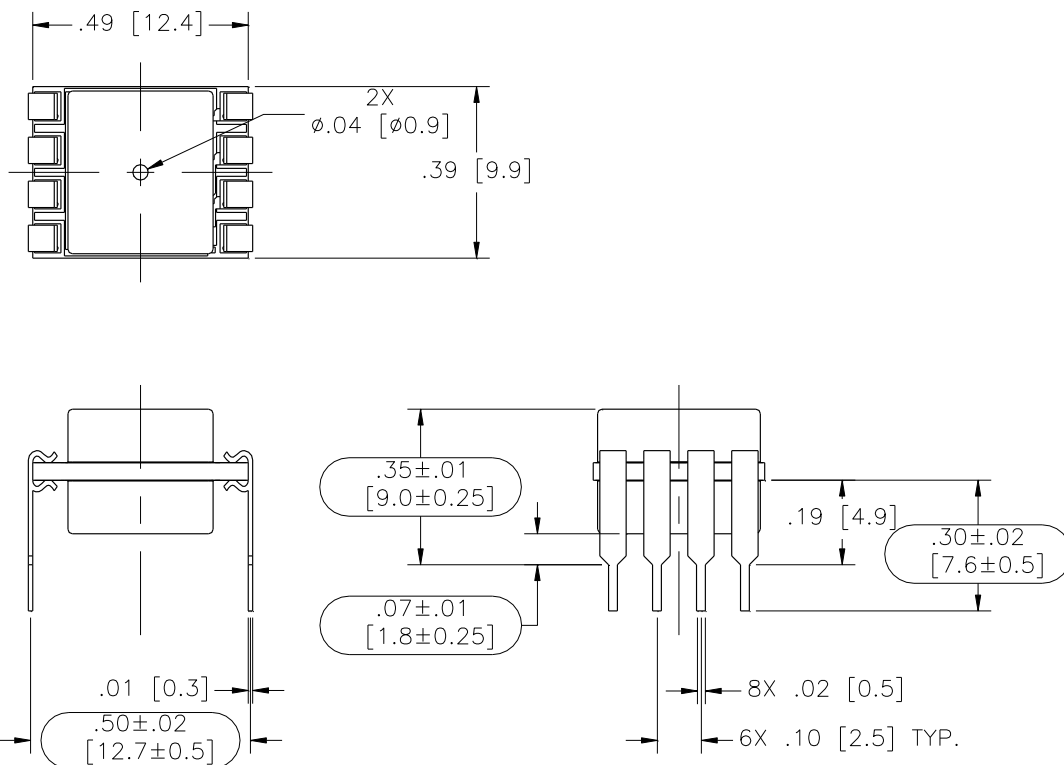
Model: MS4525-MMvoxxxP
