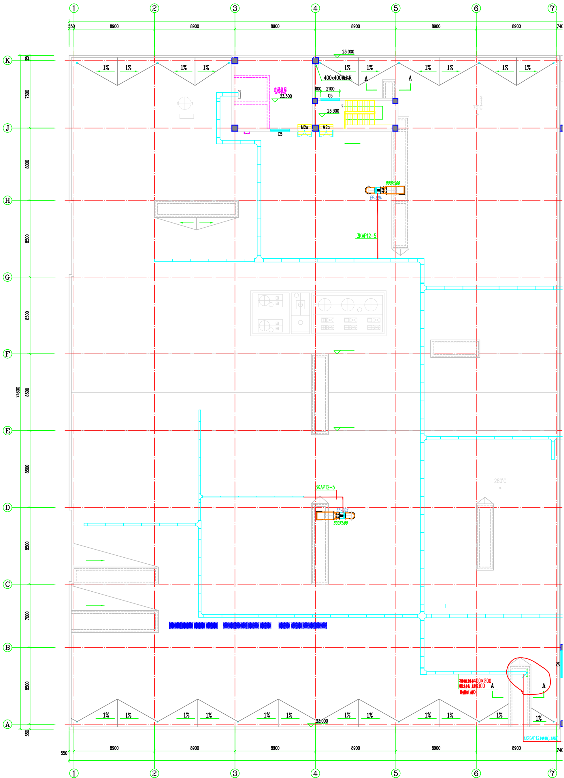
屋面空调配电平面图 1:150
