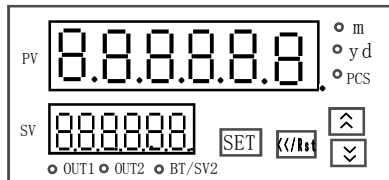
FH8 6 digit counter or length
