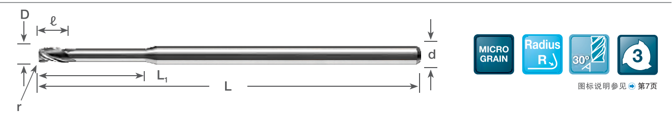
标准圆角延长刃(英制规格)
