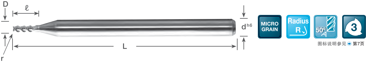
大螺旋角圆角标准刃(英制规格)
