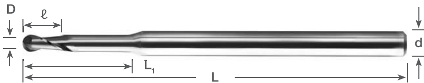
延长刃(公制规格)
