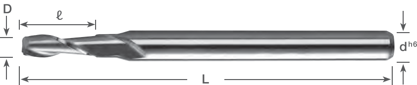
标准刃(公制规格)
