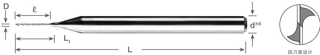
标准刃长
